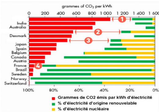
Facteurs d'émissions de la production électrique dans le monde.
